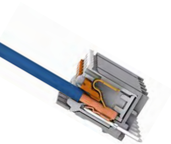
picoMAX® konnektör
