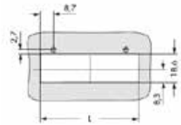
Panel geçiş yuvası şase punch değerleri
