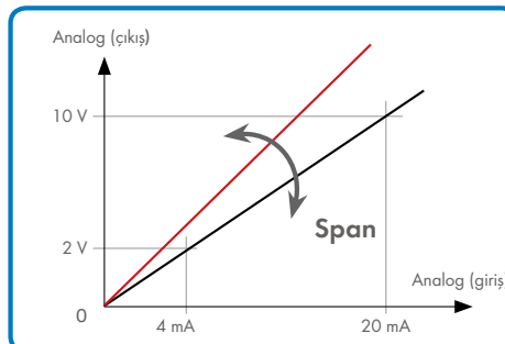
Span-Ayarı
