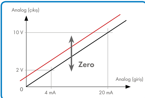
Zero-Ayarı
