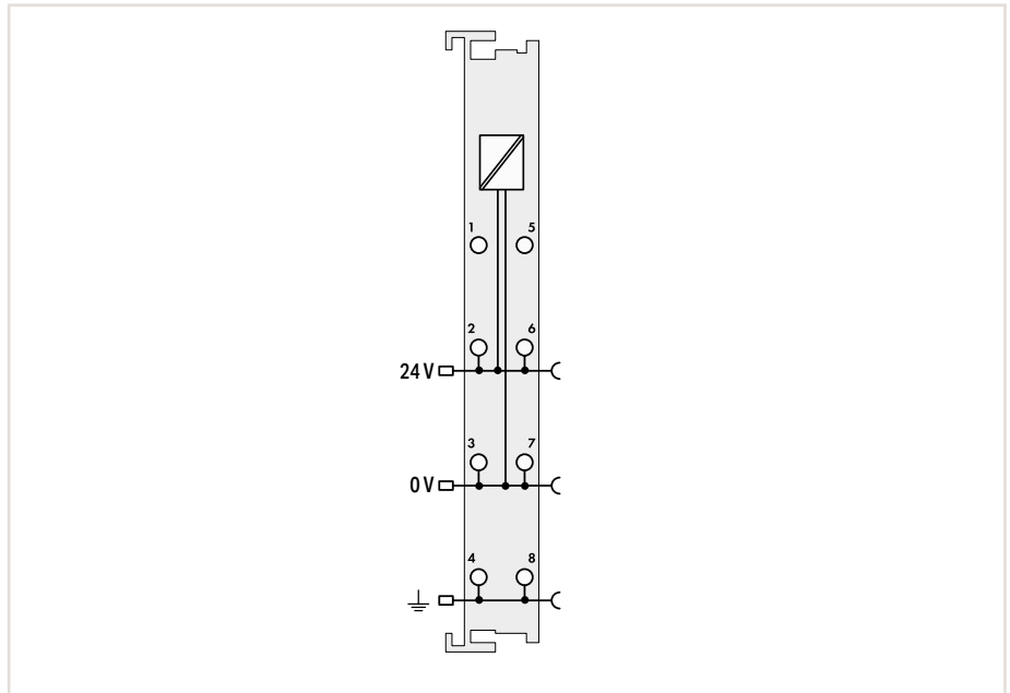
Figure: 750-624/020-000
