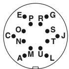
M16 geçmeli bağlantı için konnektör pin ataması, 14-pinli
