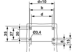
Pano kesiji
