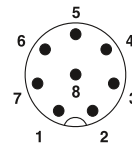
M12 geçmeli bağlantı için konnektör pin ataması, 8-pinli
