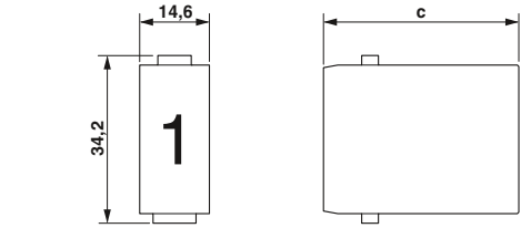
1 modül slotu
