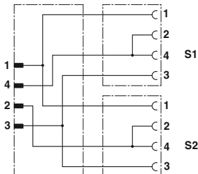
M12 fiş ve M12 soketin kontak ataması, köprülü
