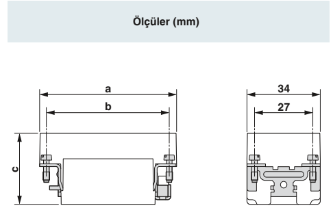
Boyutlu çizim
