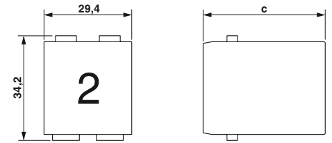
2 modül slotu
