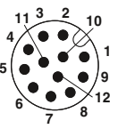
M12 geçmeli bağlantının pin dağılımı, 12 pinli
