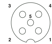
M12 soketin pin ataması, 5-kut.
